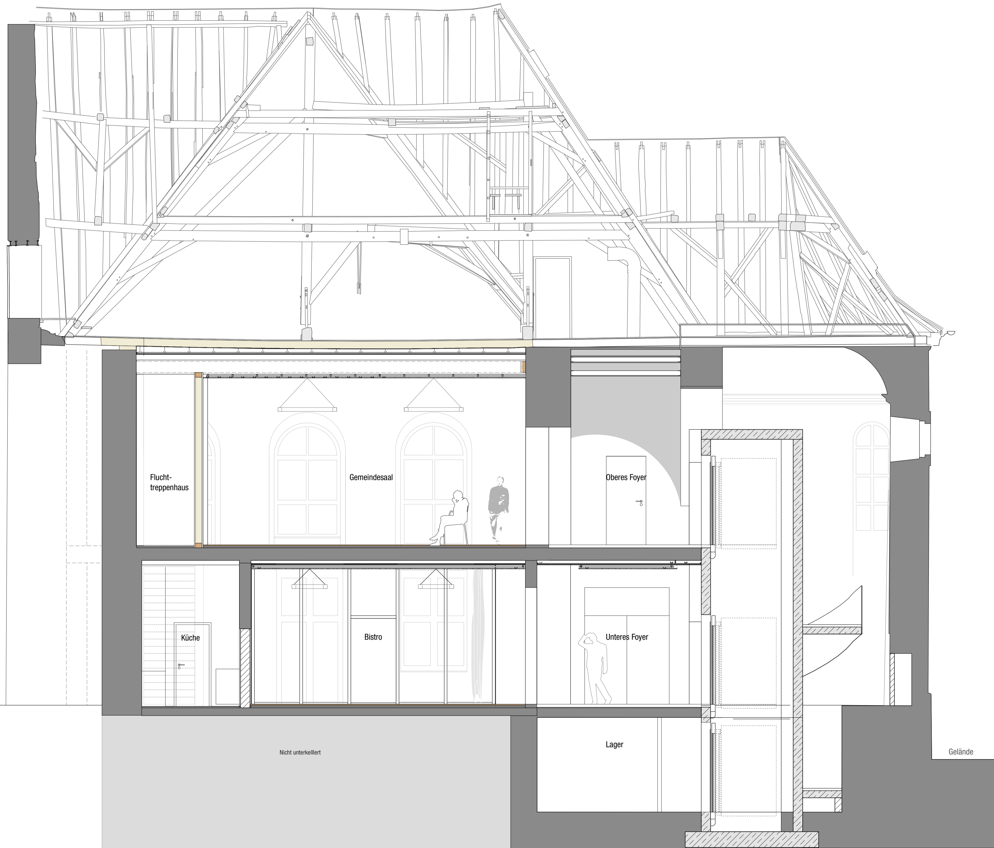
Schnitt A-A
