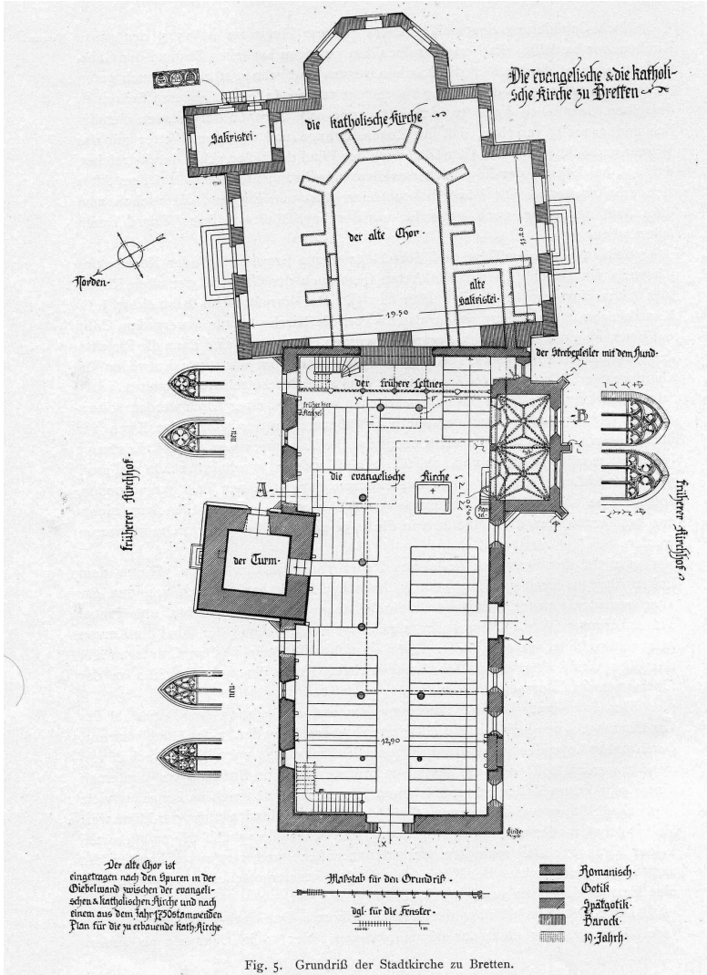
Fig. 5. Grundriß der Stadtkirche zu Bretten.
